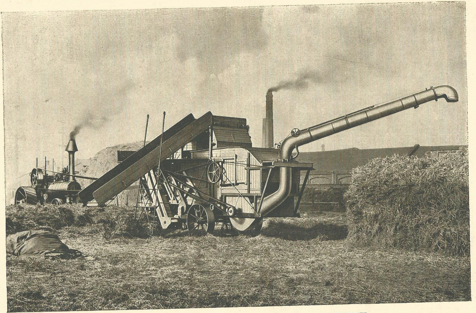
CLAYTON & SHUTTLEWORTH'S ARGENTINISCHE DRESCHGARNTUR IN ARBEIT.
